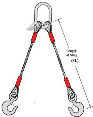
2 Leg Redi-Grip® Sling
