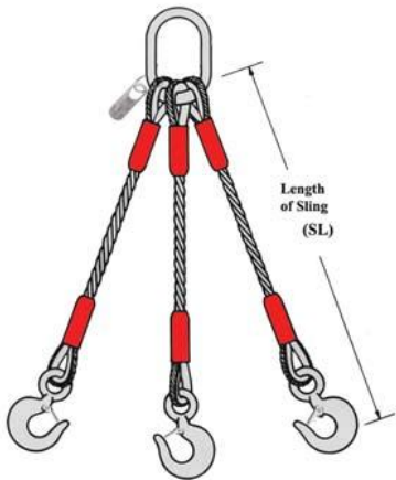
3 Leg Redi-Grip® Sling
